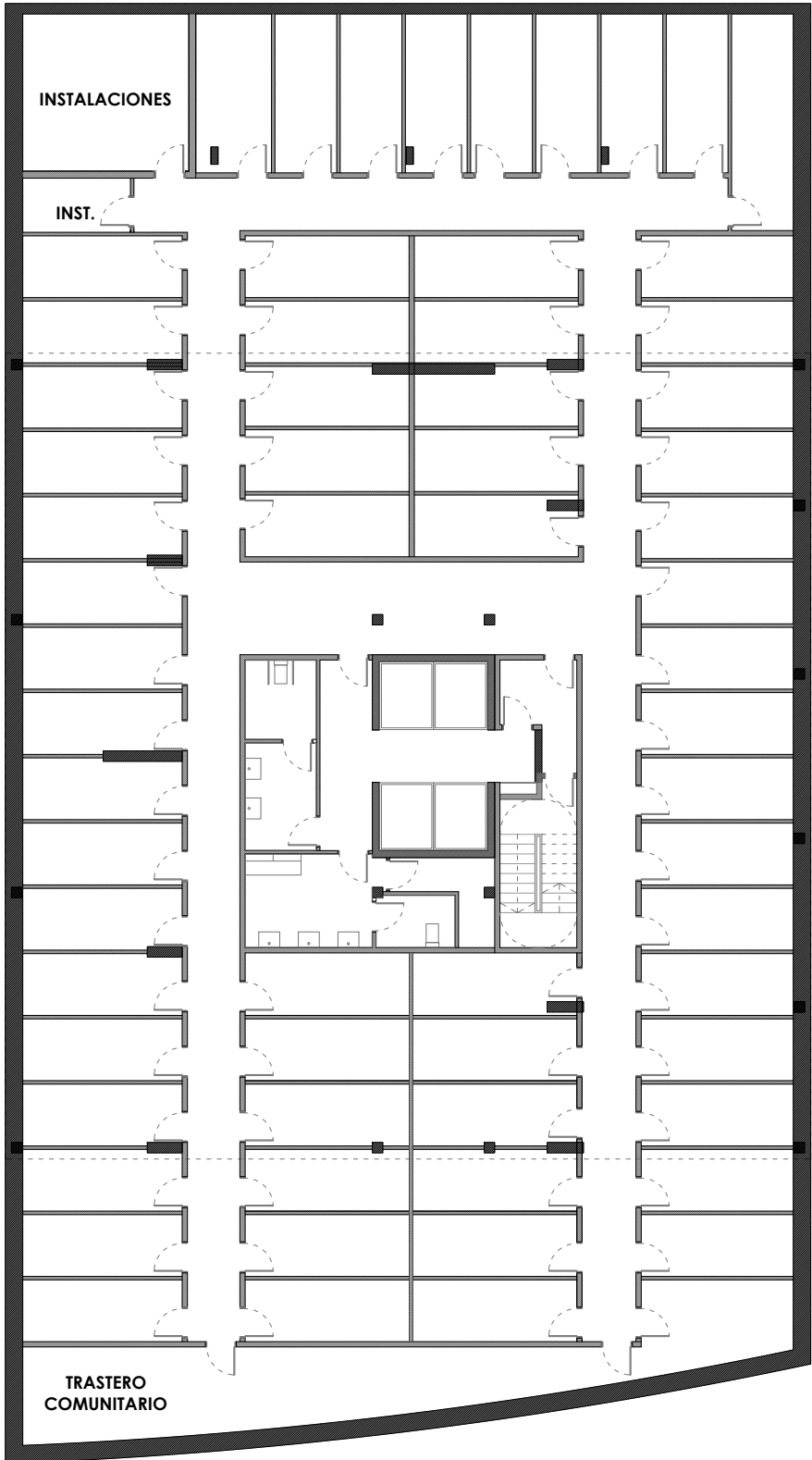
SÓTANO -4 TRASTEROS
