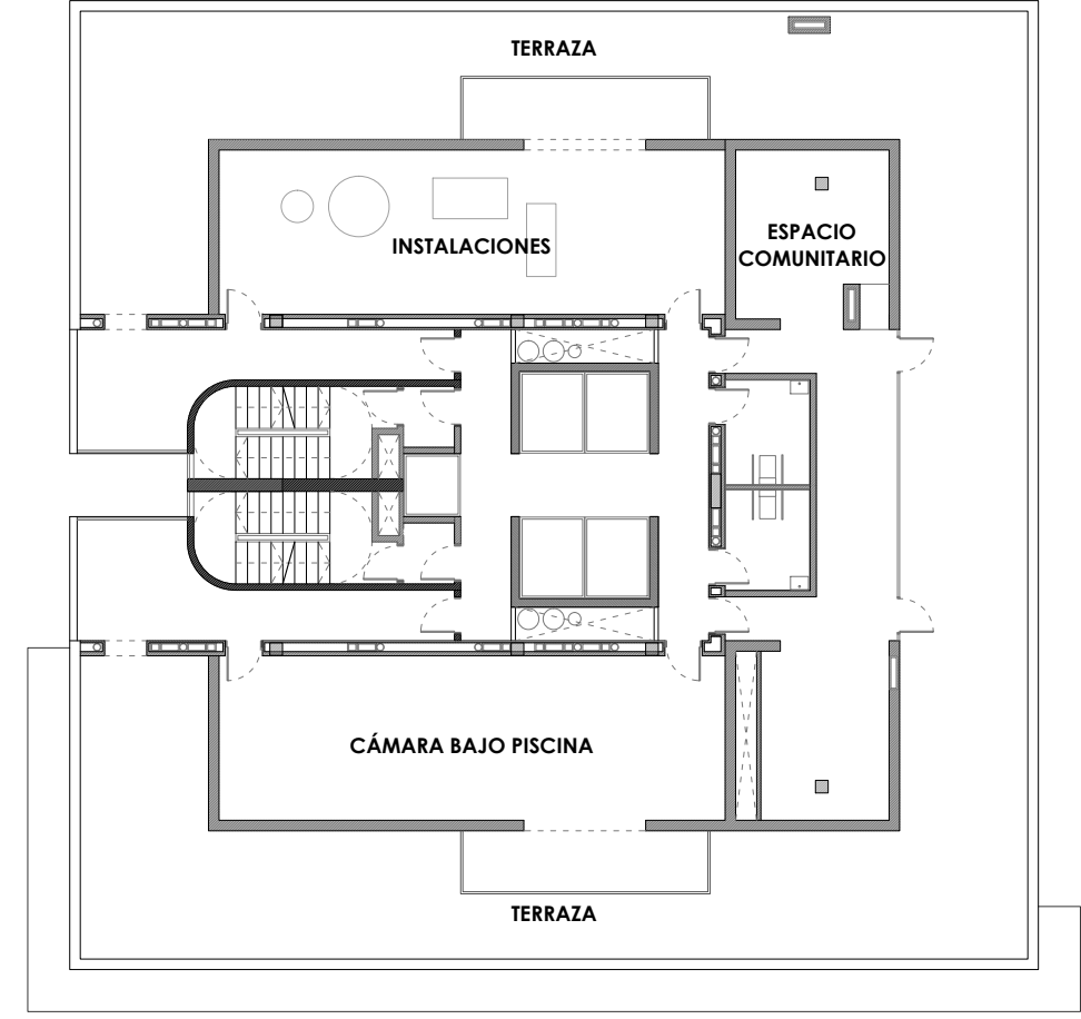
PLANTA ÁTICO
